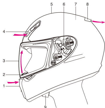
Upper Air Intake / Prise d'air supérieure
