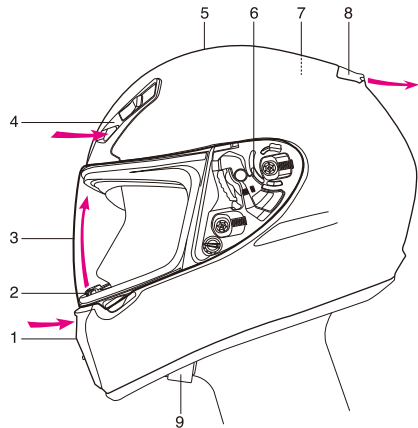
Ylempi ilmanottoaukko / Övre luftintag
